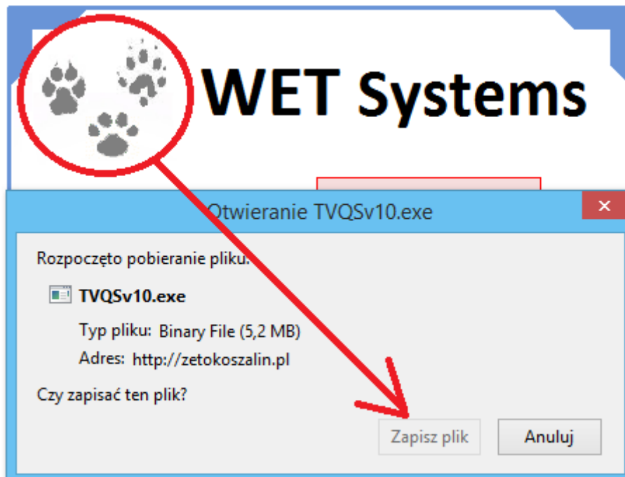
Rysunek 7 TeamViewer
